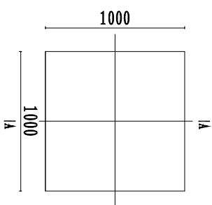
乔木种植穴大样(一) 1:25
