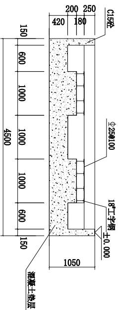
B-B剖面图
