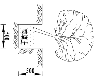
灌木栽植图示 单位: mm
