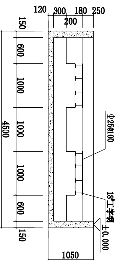
A-A剖面图
